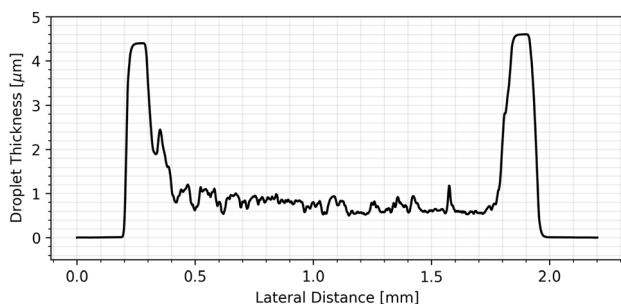
(b) \text{Cs}_3\text{Bi}_2\text{Br}_9\text{-Cs}_3\text{Sb}_2\text{I}_9 Droplet Thickness Profile
