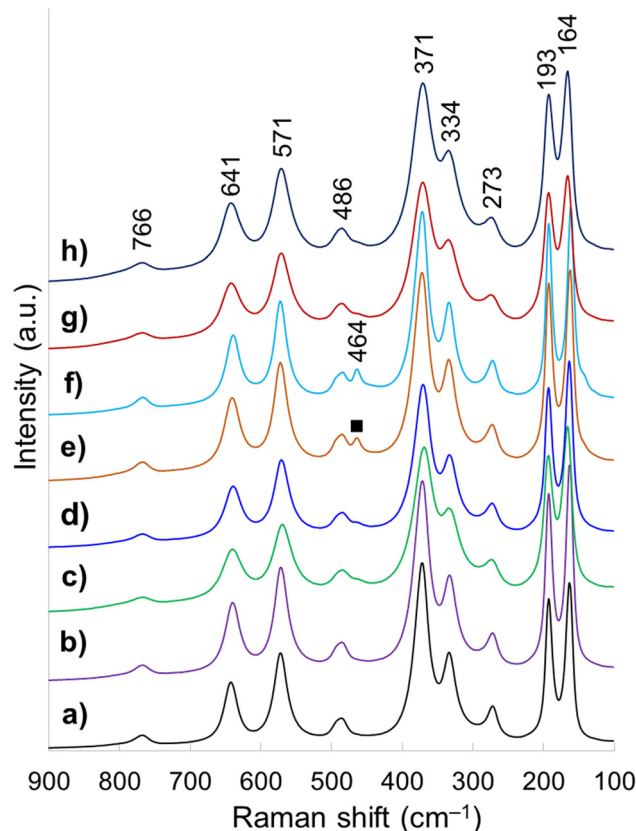
Fig. 3 Raman spectra of samples (a) w0, (b) \phi 12w1-4, (c) \phi 12w1-2, (d) \phi 12w3-4, (e) \phi 8w1-2, (f) \phi 8w3-4, (g) \phi 20w1-2, (h) \phi 20w3-4, (■) CeO 2 .
