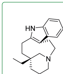
132 : (-)-Quebrachamine
