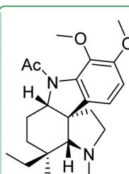
133 : (-)-Pyrifolidine
