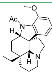
134 : (-)-Aspidospermine
