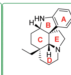
135 : (+)-Aspidospermidine
