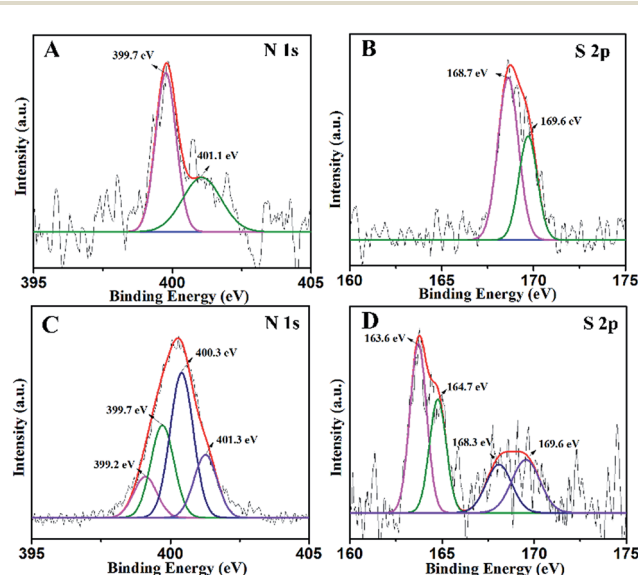
Fig. 4 High-resolution N 1s XPS spectra of (A) NST and (C) NSTG(1 : 3) and S 2p of (B) NST and (D) NSTG(1 : 3).
