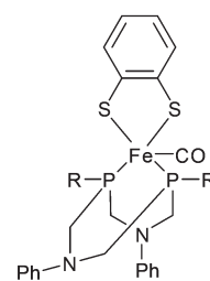
[Fe( \mu -bdt)(CO) P^R_2N^{Ph}_2 ]
