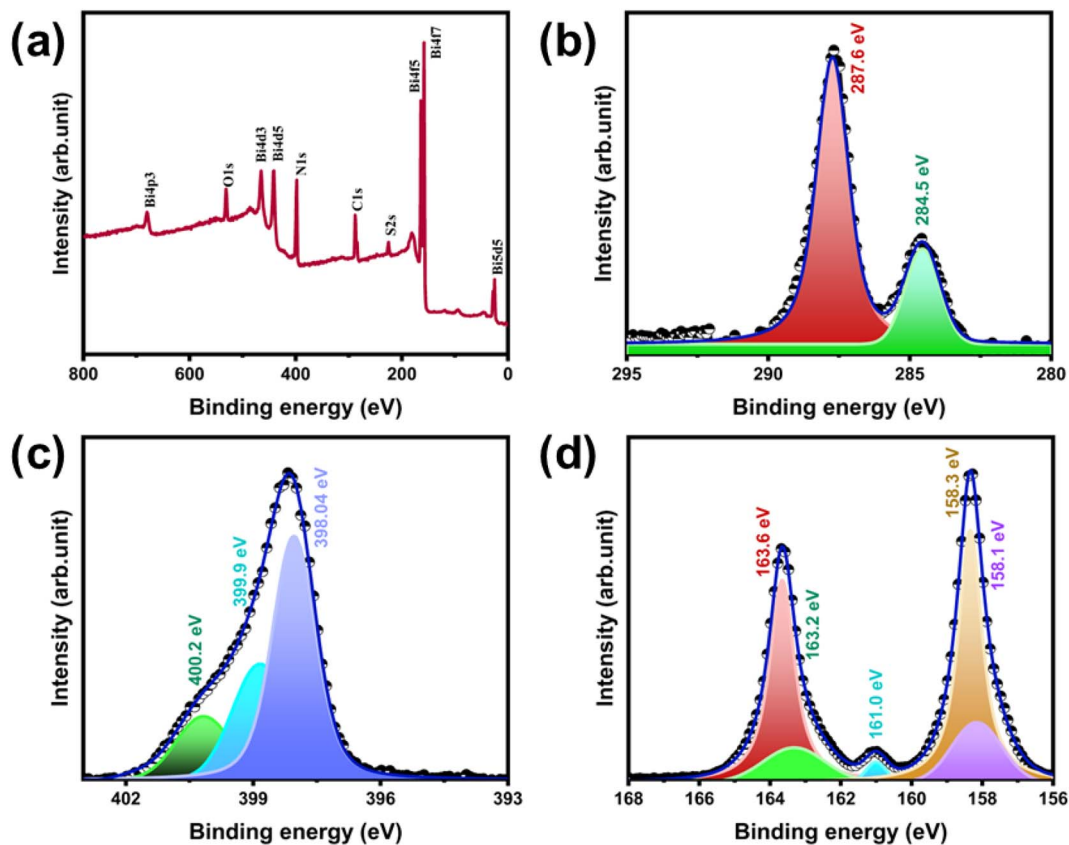
Fig. 4 XPS (a) survey scan of g\text{-C}_3\text{N}_4/\text{Bi}_2\text{S}_3 foam. (b)–(d) Narrow scan XPS of g\text{-C}_3\text{N}_4/\text{Bi}_2\text{S}_3 foam: (b) C 1s and (c) N 1s and (d) Bi 4f.
