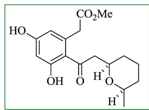
624: Curvulone B
