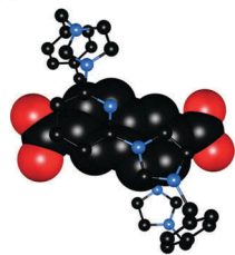
(d) \text{100} \cdot (\text{103})_3 \cdot \text{Ag}_2 \cdot 16\text{H}_2\text{O} - polyrotaxane
