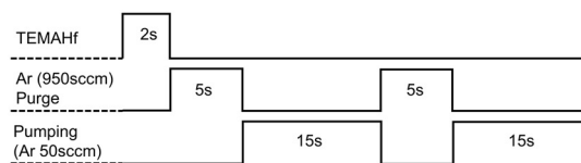
(d) Main ALD step
