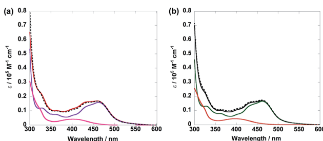
Fig. 1 UV-vis absorption spectra of (a) Ru(CH 2 OCH 2 )Re (red), Ru(CH 2 OCH 2 ) (purple), and Re(CH 2 OCH 2 ) (pink), and Ru(CH 2 OCH 2 ) + Re(CH 2 OCH 2 ) (black), Ru (green), and Re (red). The dotted lines show the 1:1 summation spectrum of (a) Ru(CH 2 OCH 2 ) and Re(CH 2 OCH 2 ) and (b) Ru and Re . Dimethylformamide (DMF) was used as the solvent.
