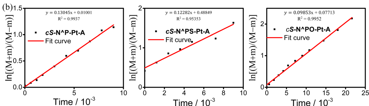
Fig. 8 (a) X-ray single-crystal structures, dihedral angles, and experimental interconversion energy barriers of cS-N1 A O-Pt-A , cS-N2 A O-Pt-B , cS-N A P-Pt-A , cS-N A PO-Pt-A , and cS-N A PS-Pt-A ; (b) investigation of rotation barriers of cS-N A P-Pt-A , cS-N A PO-Pt-A , and (cS)N A PS-Pt-A .
