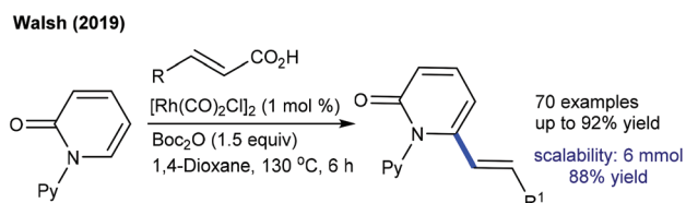
Scheme 33 Decarbonylative C–H alkenylation of pyridones.
