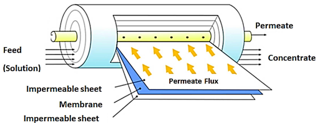
Fig. 15 Membrane filtration. 139
