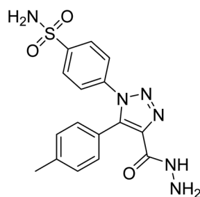
4-[4-(Hydrazinocarbonyl)-5-(p-tolyl)-1H-1,2,3-triazol-1-yl]benzenesulfonamide
