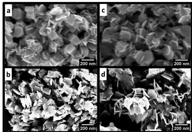
Fig. 3 SEM images of (a) WO 3 _180 °C-0 min, (b) WO 3 _200 °C-0 min, (c) WO 3 GO_180 °C-0 min and (d) WO 3 GO_200 °C-0 min.
