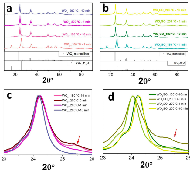
Fig. 4 XRD of (a) WO 3 _180 °C-1 min, WO 3 _180 °C-10 min, WO 3 _200 °C-1 min, WO 3 _200 °C-10 min and (b) WO 3 GO_180 °C-1 min, WO 3 GO_200 °C-1 min, WO 3 GO_200 °C-10 min. Magnified XRD region between 23 and 26° of (c) WO 3 _180 °C-10 min, WO 3 _200 °C-0 min, WO 3 _200 °C-1 min, WO 3 _200 °C-10 min and (d) WO 3 GO_180 °C-10 min, WO 3 GO_200 °C-0 min, WO 3 GO_200 °C-1 min and WO 3 GO_200 °C-10 min.
