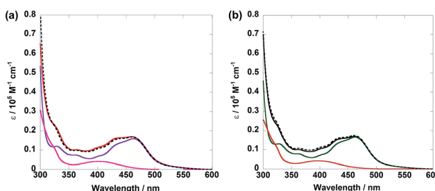
Fig. 1 UV-vis absorption spectra of (a) Ru(CH 2 OCH 2 )Re (red), Ru(CH 2 OCH 2 ) (purple), and Re(CH 2 OCH 2 ) (pink), and Ru(CH 2 CH 2 CH 2 )Re (black), Ru (green), and Re (red). The dotted lines show the 1:1 summation spectrum of (a) Ru(CH 2 OCH 2 ) and Re(CH 2 OCH 2 ) and (b) Ru and Re . Dimethylformamide (DMF) was used as the solvent.
