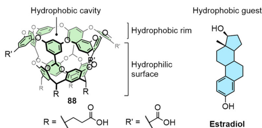
Estradiol
