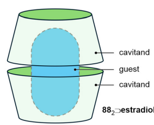
Estradiol
