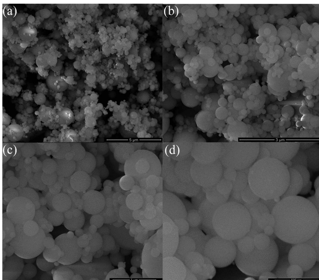
Fig. 2 Scanning electron microscope of fly ash cenosphere in different scales: (a) 20 000×, (b) 50 000×, (c) 10 000×, (d) 2 000×.
