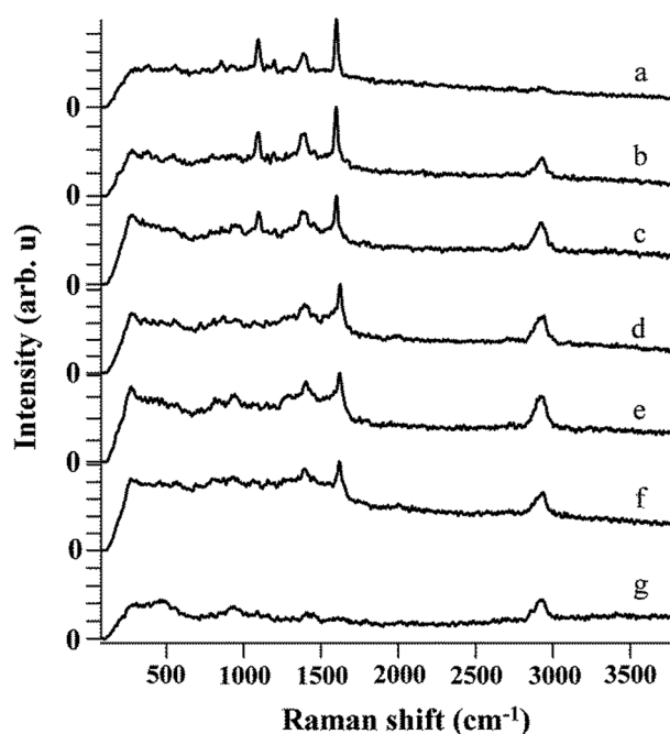
Fig. 5 SERS spectrum of MBA on SERS substrate with concentrations of (a) 10^{-3} M, (b) 10^{-5} M, (c) 10^{-7} M, (d) 10^{-9} M, (e) 10^{-11} M, (f) 10^{-13} M, (g) 0 M.
