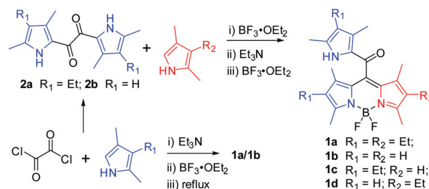
Scheme 1 Syntheses of meso -2-ketopyrrolyl BODIPYs 1a–d .
