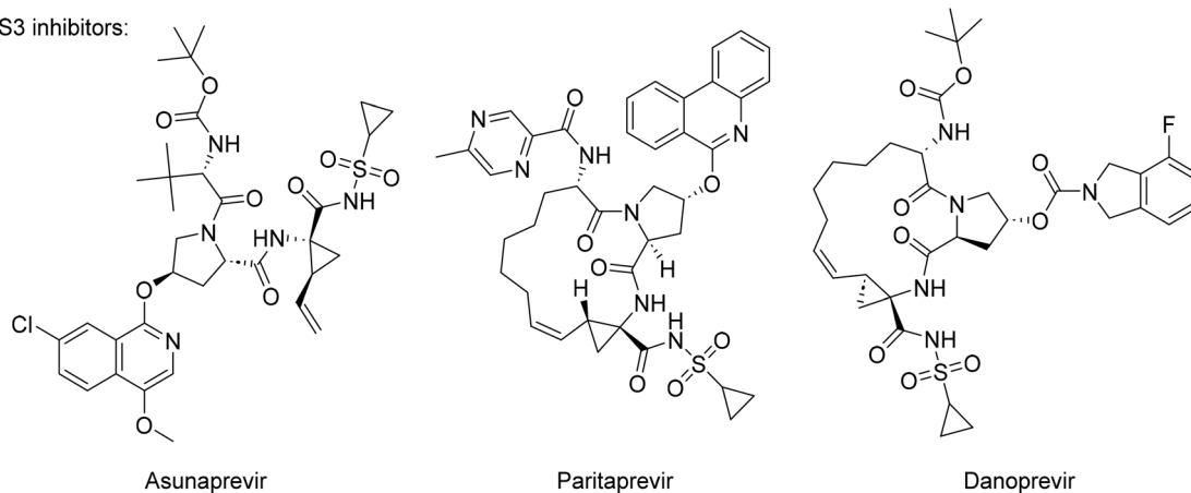
Asunaprevir
