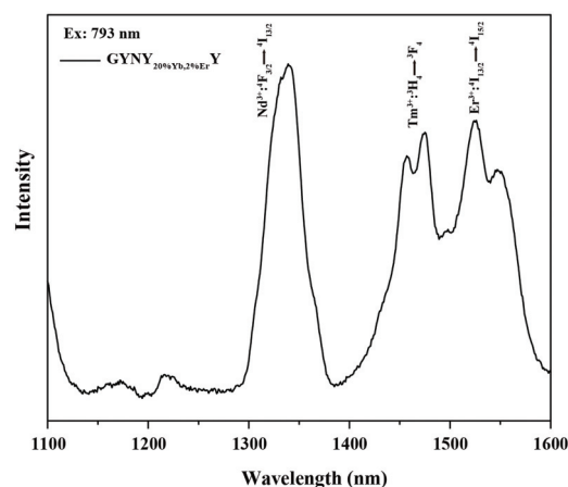
Fig. 2 Downshifting emission spectrum of \text{NaGdF}_4\text{:}49\%\text{Yb}, 1\%\text{Tm}@ \text{NaYF}_4\text{:}20\%\text{Yb}@ \text{NaNF}_4\text{:}10\%\text{Yb}@ \text{NaYF}_4\text{:}20\%\text{Yb}, 2\%\text{Er}@ \text{NaYF}_4 nanocrystals.
