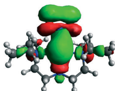
(c) [Pd(Bu4dien)(NO 2 )] + (reference 38)
