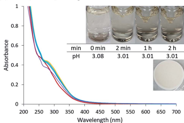
(b) BBOA (Pine #2) + FeCl 3
