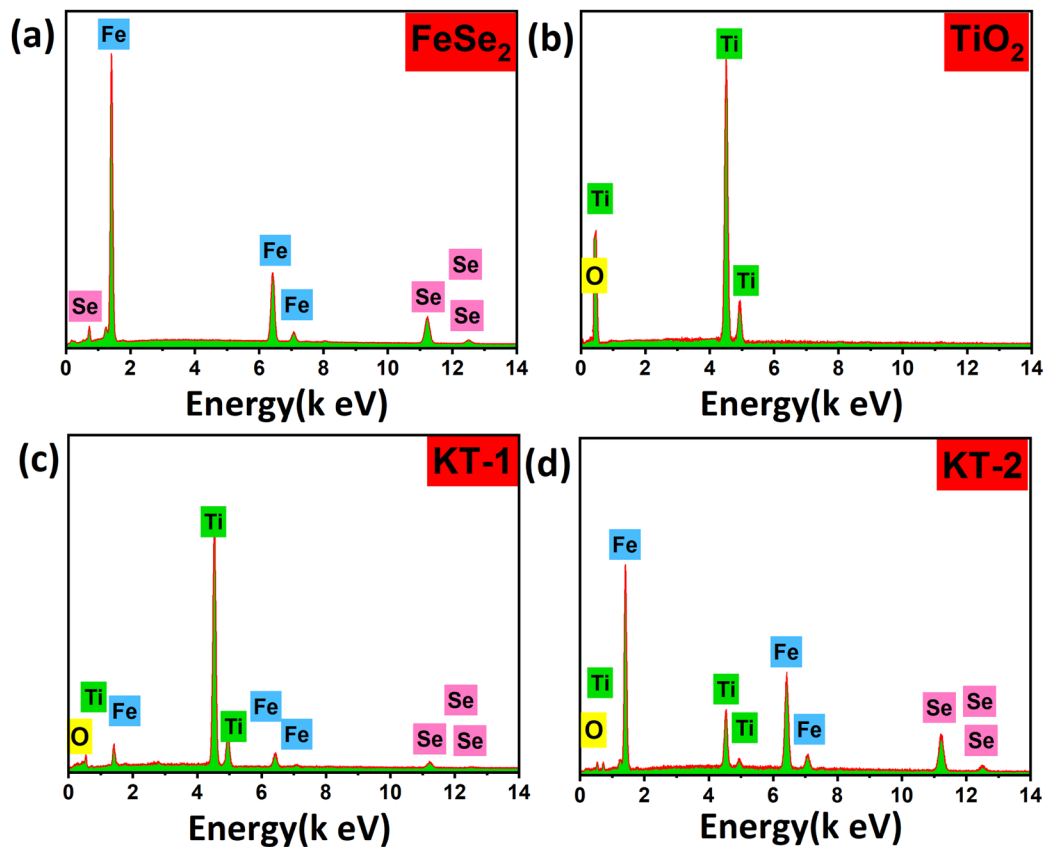
Fig. 3 EDX of (a) \text{FeSe}_2 and (b) \text{TiO}_2 , and (c) \text{KT-1} (d) \text{KT-2} composites.
