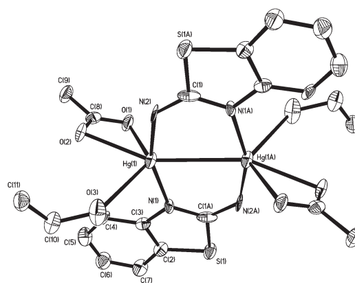
Fig. 1 Molecular structure of 3 . Thermal ellipsoids are displayed at 50% probability and hydrogen atoms omitted for clarity. Selected bond lengths (Å) and bond angles ( ^\circ ): \text{Hg}1-\text{Hg}1\text{A} 3.094(1), \text{Hg}1-\text{N}1 2.067(6), \text{Hg}1-\text{N}2 2.040(8), \text{Hg}1-\text{O}1 2.560(7), \text{Hg}1-\text{O}2 2.481(6), \text{Hg}1-\text{O}3 2.592(8), \text{N}1-\text{C}1\text{A} 1.348(11), \text{N}2-\text{C}1 1.286(10), \text{C}1-\text{S}1\text{A} 1.738(8); \text{N}1\text{A}-\text{C}1-\text{N}2 126.5(7), \text{N}1-\text{Hg}-\text{N}2 158.5(2), \text{O}1-\text{Hg}-\text{O}2 114.5(2), \text{N}1-\text{Hg}1-\text{O}3 91.1(2).
