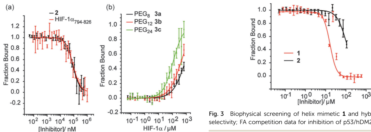
3 = FITC-Ahx-QLTSYDCEVNA-(PEG) x -EELLRALDQVN-NH 2
