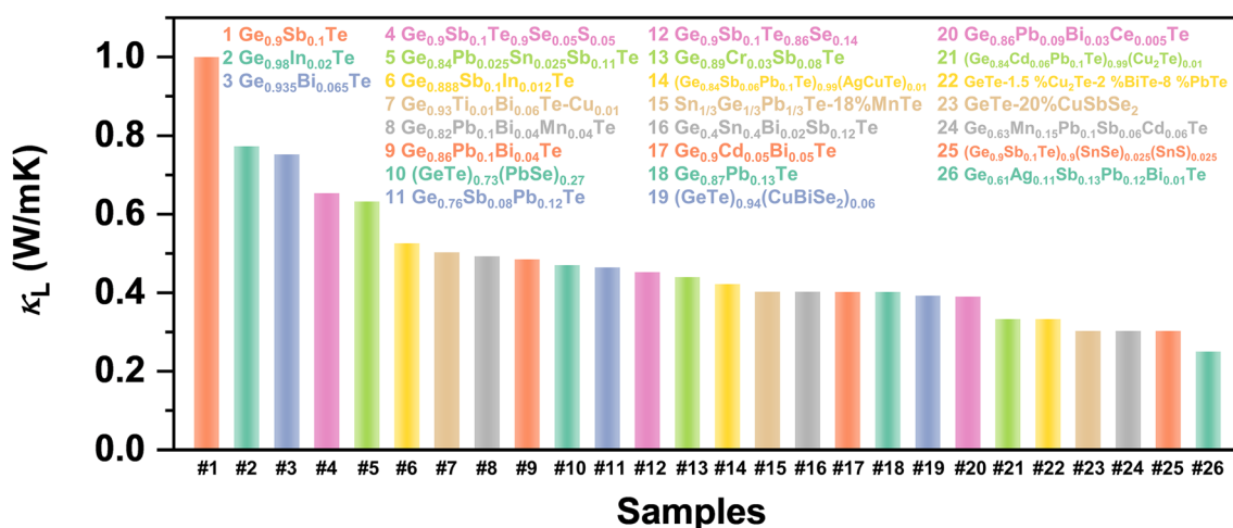
Fig. 15 Summary of reported minimum lattice thermal conductivity in Ge 0.9 Sb 0.1 Te, 19 Ge 0.98 In 0.02 Te, 125 Ge 0.935 Bi 0.065 Te, 18 Ge 0.9 Sb 0.1 Te 0.95 Se 0.05 Sb 0.05 , 17 Ge 0.84 Pb 0.025 Sn 0.025 Sb 0.11 Te, 45 Ge 0.888 Sb 0.1 In 0.012 Te, 23 Ge 0.93 Ti 0.01 Bi 0.06 Te-Cu 0.01 , 134 Ge 0.82 Pb 0.1 Bi 0.04 Mn 0.04 Te, 37 Ge 0.86 Pb 0.1 Bi 0.04 Te, 25 (GeTe) 0.73 (PbSe) 0.27 , 113 Ge 0.76 Sb 0.08 Pb 0.12 Te, 21 Ge 0.9 Sb 0.1 Te 0.86 Se 0.14 , 19 Ge 0.89 Cr 0.03 Sb 0.08 Te, 128 (Ge 0.84 Sb 0.06 Pb 0.1 Te) 0.99 (AgCuTe) 0.01 , 160 Sn 1/3 Ge 1/3 Pb 1/3 Te-18% MnTe, 161 Ge 0.4 Sn 0.4 Bi 0.02 Sb 0.12 Te, 162 Ge 0.9 Cd 0.05 Bi 0.05 Te, 22 Ge 0.87 Pb 0.13 Te, 11 (GeTe) 0.94 (CuBiSe 2 ) 0.06 , 163 Ge 0.86 Pb 0.05 Bi 0.03 Ce 0.005 Te, 164 (Ge 0.84 Cd 0.06 Pb 0.1 Te) 0.99 (Cu 2 Te) 0.01 , 50 GeTe-1.5% Cu 2 Te-2% BiTe-8% PbTe, 51 GeTe-20% CuSbSe 2 , 49 Ge 0.63 Mn 0.15 Pb 0.1 Sb 0.06 Cd 0.06 Te, 36 (Ge 0.9 Sb 0.1 Te) 0.9 (SnSe) 0.025 (SnS) 0.025 , 165 and Ge 0.61 Ag 0.11 Sb 0.13 Pb 0.12 Bi 0.01 Te. 38
