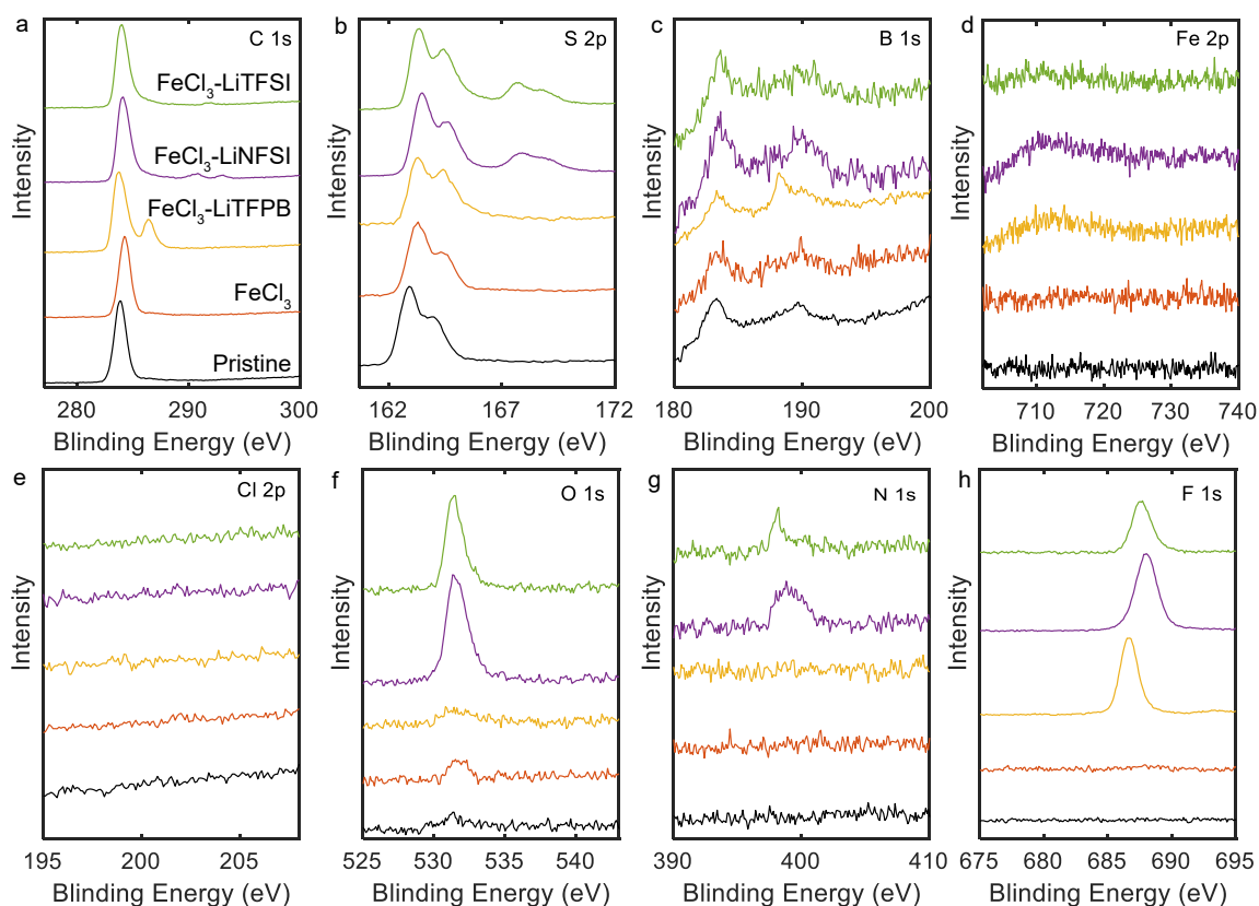
Fig. 2 XPS spectra of doped PQT thin films. (a) C 1s, (b) S 2p, (c) B 1s, (d) Fe 2p, (e) Cl 2p, (d) O 1s, (e) N 1s, and (f) F 1s regions.
