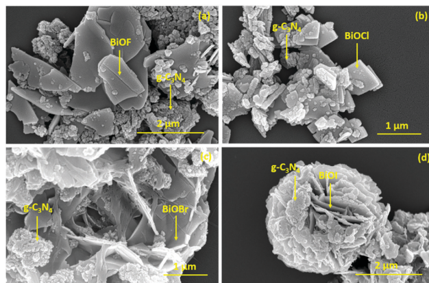
Fig. 4 FESEM images of (a) \text{BiOF}/\text{g-C}_3\text{N}_4 , (b) \text{BiOCl}/\text{g-C}_3\text{N}_4 , (c) \text{BiOBr}/\text{g-C}_3\text{N}_4 and (d) \text{BiOI}/\text{g-C}_3\text{N}_4 composites.
