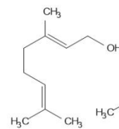
Citronellol
