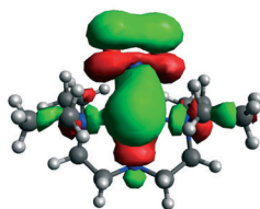
HOMO
