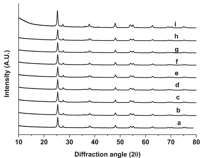
Fig. 2 XRD patterns of (a) TiO 2 P25 (b) 5% Ru/TiO 2 (c) 4% Ru–1% Pd/TiO 2 , (d) 3% Ru–2% Pd/TiO 2 , (e) 2.5% Ru–2.5% Pd/TiO 2 , (f) 2% Ru–3% Pd/TiO 2 , (g) 1% Ru–4% Pd/TiO 2 , (h) 0.5% Ru–4.5% Pd/TiO 2 , (i) 5% Pd/TiO 2 .
