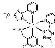
57: R = H Ir(fppz) 2 (bdp)
