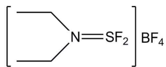
XtalFluor-E
