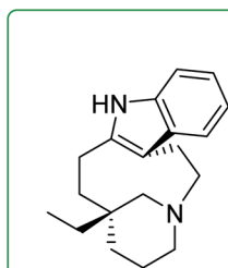
132 : (-)-Quebrachamine
