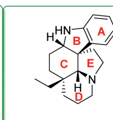
135 : (+)-Aspidospermidine
