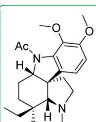
133 : (-)-Pyrifolidine
