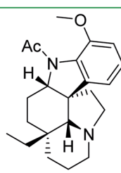
134 : (-)-Aspidospermine
