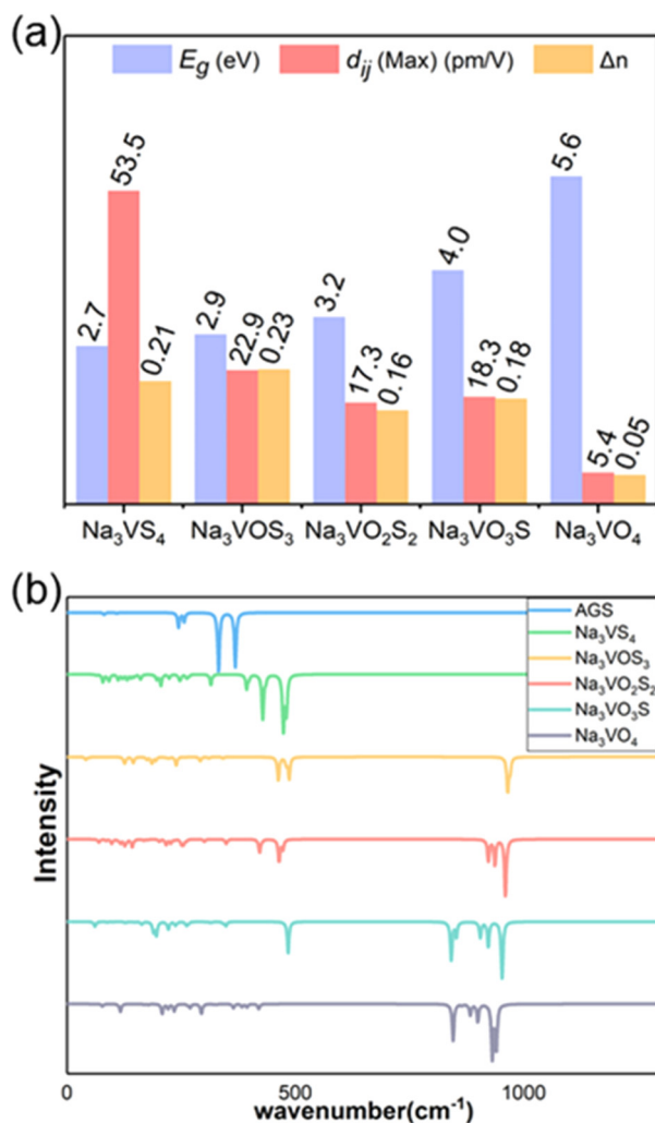
Fig. 4 (a) Band gap E g , largest SHG coefficient d ij (Max), birefringence Δ n ; (b) IR spectra of Na 3 VS 4 , Na 3 VOS 3 , Na 3 VO 2 S 2 , Na 3 VO 3 S, and Na 3 VO 4 .
