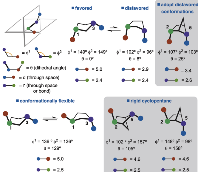
Fig. 1 Bicyclo[2.1.1]hexanes.
