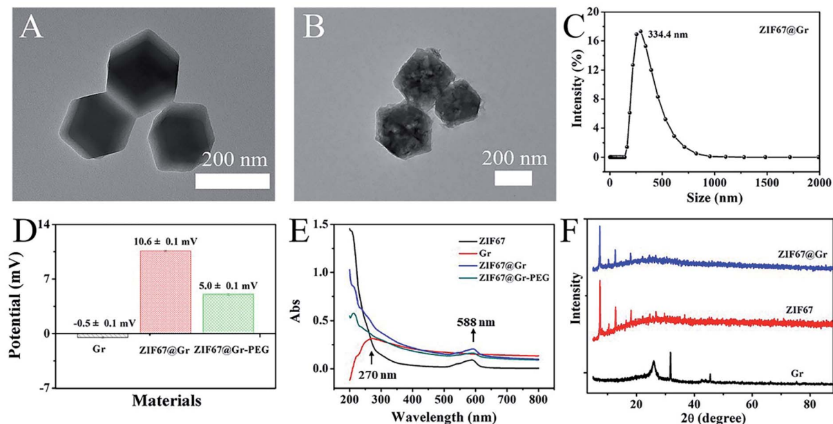
Fig. 1 Characterization of ZIF67@Gr-PEG. TEM images of (A) ZIF67 NCs and (B) ZIF67@Gr NCs. The scale bar is 200 \mu m. (C) Hydrodynamic diameter of ZIF67@Gr. (D) Zeta potentials of Gr, ZIF67@Gr and ZIF67@Gr-PEG. (E) UV-vis spectra of Gr, ZIF67, ZIF67@Gr and ZIF67@Gr-PEG. (F) XRD patterns of Gr, ZIF67, and ZIF67@Gr.
