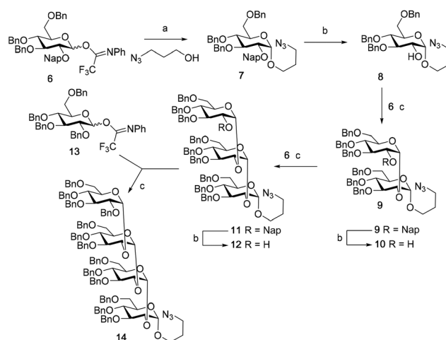
Scheme 2 The assembly of kojiligosaccharides. (a) TMSI, \text{Ph}_3\text{P}=\text{O} , DCM, 36 h, 75%, \alpha : \beta = 10 : 1 . (b) DDQ, \text{DCM} : \text{H}_2\text{O} = 10 : 1 (v : v), 8 : 75%; 10 : 49%; 12 : 47%. (c) DMF, TfOH, DCM, 9 : 95%, \alpha : \beta = 15 : 1 ; 11 : 67%, \alpha : \beta = 10 : 1 ; 14 : 67%, \alpha : \beta = 2 : 1 .
