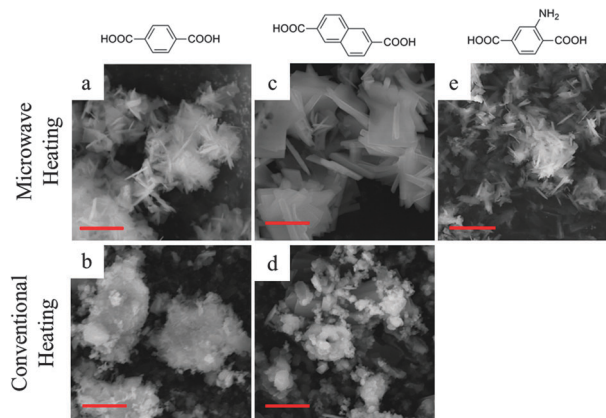
Fig. 2 SEM images of (a) MIL-140A-MW, (b) MIL-140A-CE, (c) MIL-140B-MW, (d) MIL-140B-CE and (e) MIL-140A-NH 2 -MW (scale bar = 3 \mu m).
