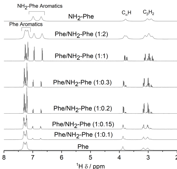
Fig. 16 ^1\text{H} solution-state NMR spectra of the Phe (303 mM), Phe/ \text{NH}_2 -Phe (1 : 0.1), Phe/ \text{NH}_2 -Phe (1 : 0.15), Phe/ \text{NH}_2 -Phe (1 : 0.2), Phe/ \text{NH}_2 -Phe (1 : 0.2), Phe/ \text{NH}_2 -Phe (1 : 0.15), Phe/ \text{NH}_2 -Phe (1 : 0.1), Phe/ \text{NH}_2 -Phe (1 : 0.3) suspension and Phe/ \text{NH}_2 -Phe (1 : 1) solution, acquired at 298 K.
