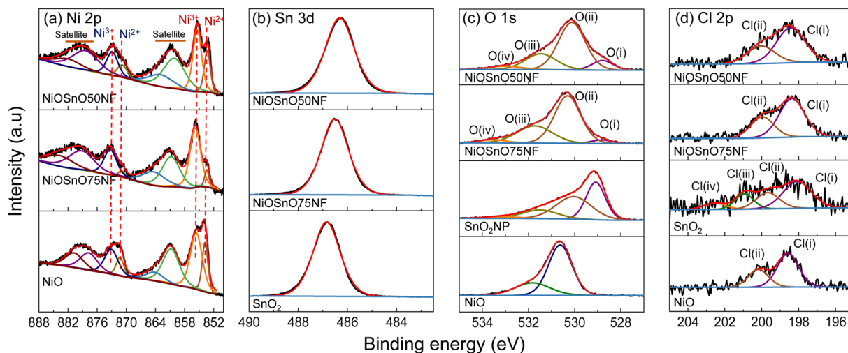
Fig. 4 (a) Ni 2p, (b) Sn 3d, (c) O 1s, and (d) Cl 2p XPS core spectra for NiOSnO50NF, NiOSnO75NF, NiO, and SnO 2 .
