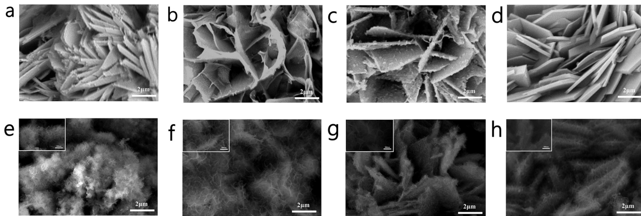
Fig. 1 SEM images of (a) \text{NCMO}_x-5 ; (b) \text{NCMO}_x-10 ; (c) \text{NCMO}_x-15 ; (d) \text{NCMO}_x-20 ; (e) \text{NCMS}_x-5 ; (f) \text{NCMS}_x-10 ; (g) \text{NCMS}_x-15 ; and (h) \text{NCMS}_x-20 .
