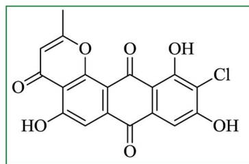
482a: Topopyrone A
