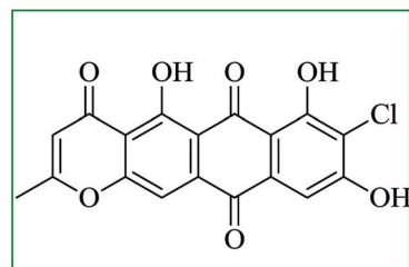
482b: Topopyrone B
