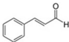
E-cinnamaldehyde
