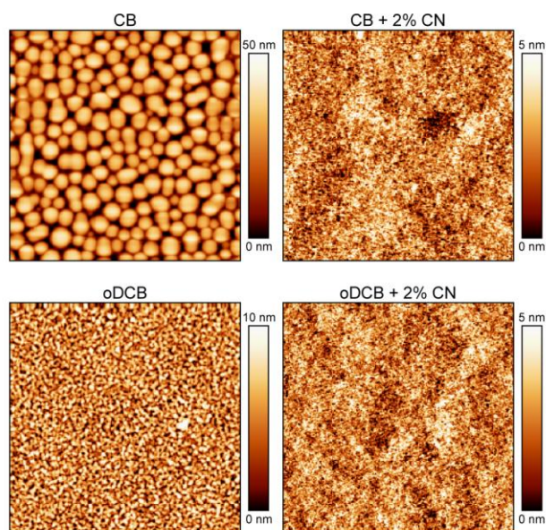
Figure 4. AFM height images ( 5 \times 5 \mu\text{m}^2 ), of TQ1:PC 70 BM 1:3 w/w, spincoated from CB, CB + 2% CN, oDCB and oDCB + 2% CN. RMS roughness values are 6.6 nm (CB), 1.3 nm (oDCB), 0.45 nm (CB + 2% CN), 0.47 nm (oDCB + 2% CN).
