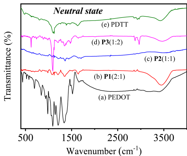
Fig. 3 FTIR spectra of (a) PEDOT, (b) P1(2 : 1), (c) P2(1 : 1), (d) P3(1 : 2) and (e) PDDT in the neutral form.
